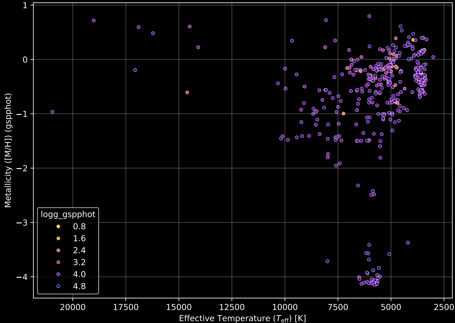
APOGEE DR17 Field: [ORIONA] Stellar Population Parameters (n= 396)
